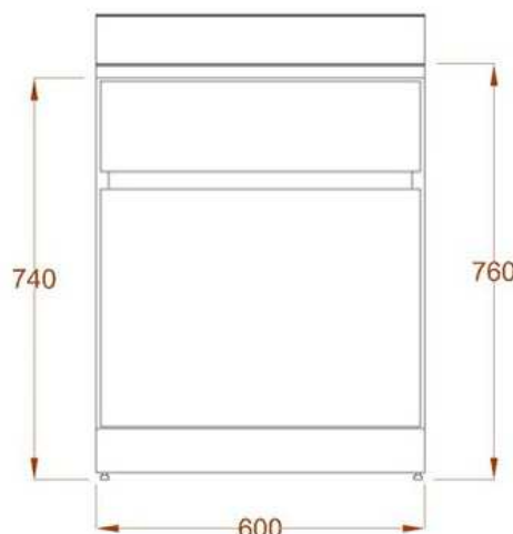
Vista frente
