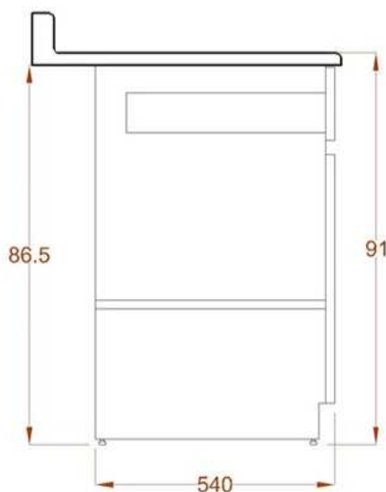
Vista lateral
